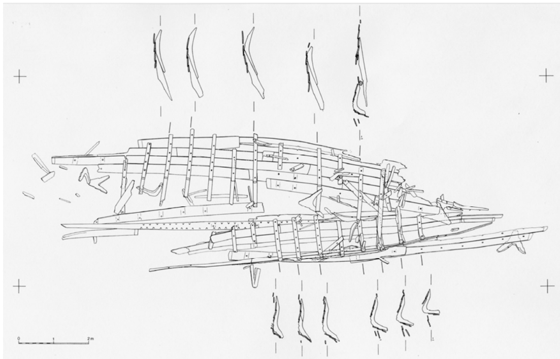
Figur 2 Plan og snit af Roskilde Havn vrug 2 (anlæg 1). Forskibet er mod højre, nord omtrent opad.
