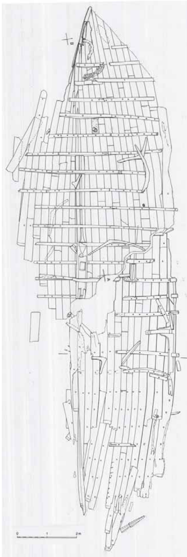
Figur 2 Udgravningsplan over Roskilde 4. Forstævnen er opad.
