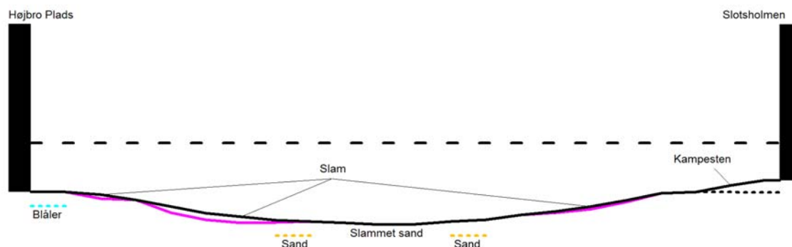
Figur 2: Tværprofil. Målestok 1:150. Opmåling: Nordic Marine Service. Med kortstiplet signatur indtegnet iagttagelser gjort ved undersøgelsen. Grafik: Mikkel H. Thomsen © Vikingskibsmuseet.
